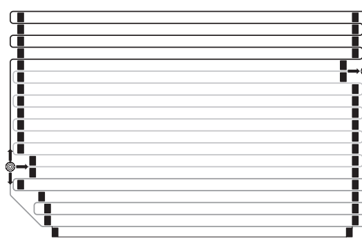
Flujo triple
